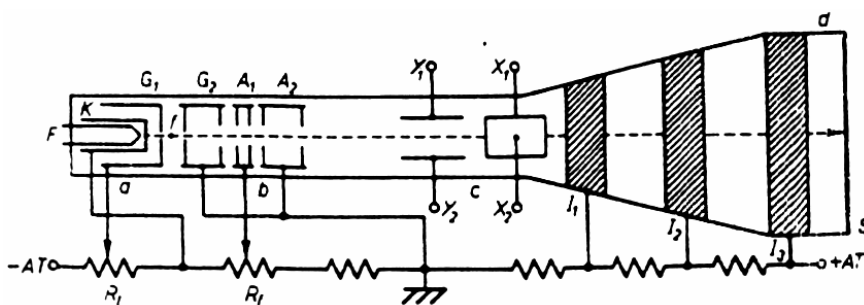
Fig. 2 - Schema del tubo a raggi catodici.
